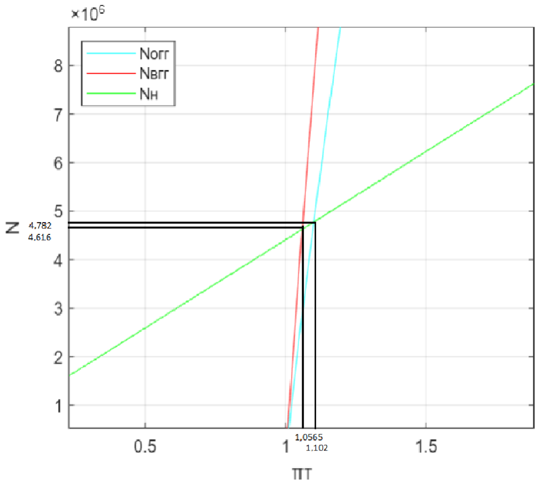
Рис. 1 Зависимость N(\pi_T) , где N_H(\pi_T) обозначен зеленым цветом, N_{ОГГ}(\pi_T) - голубым цветом, N_{ВГГ}(\pi_T) - красным цветом.
